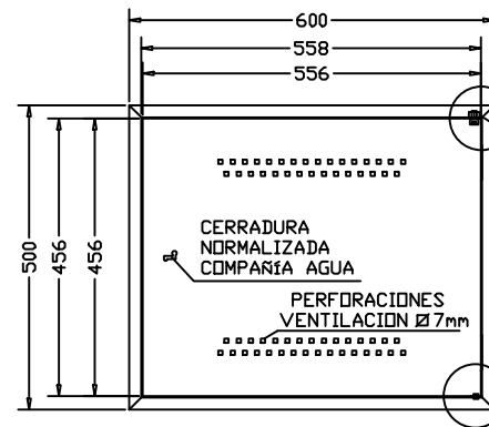
CONJUNTO
