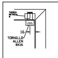
DETALLE D
