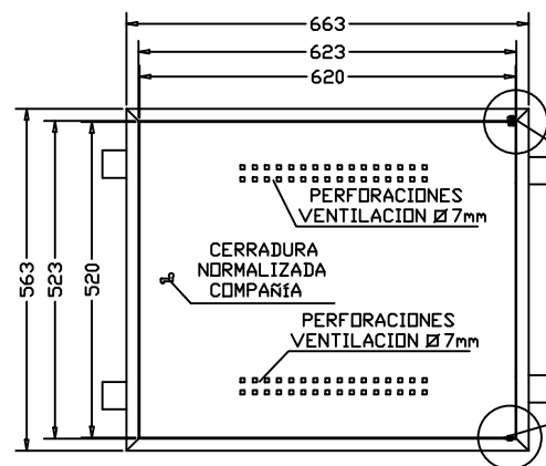
CONJUNTO
