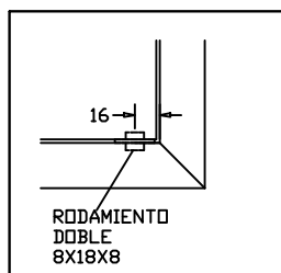
DETALLE C
