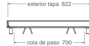
Corte B-B 1:20
