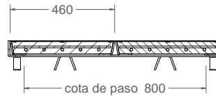
Corte A-A 1:20
