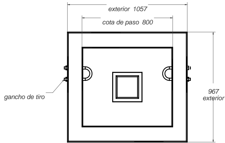
vista en planta 1:20
