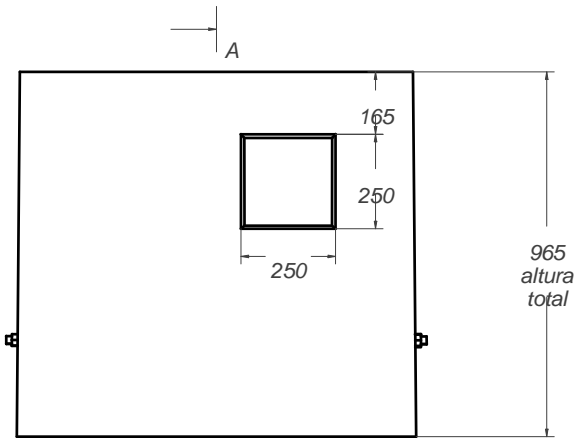
vista alzado 1:20
