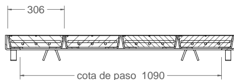
Corte A-A 1:20
