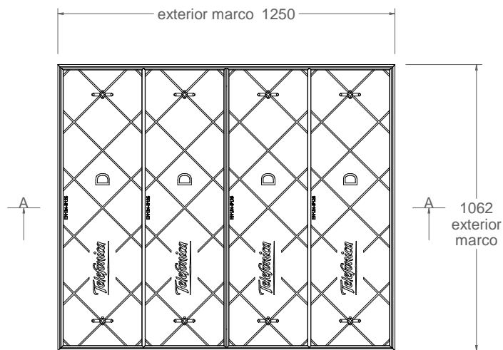
vista en planta 1:20
