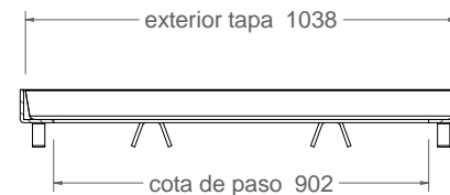
Corte B-B 1:20
