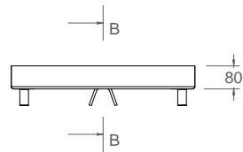
vista alzado 1:20
