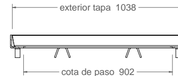
Corte B-B 1:20
