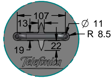
DETALLE A
